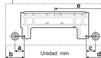
Estructura de la unidad interior
